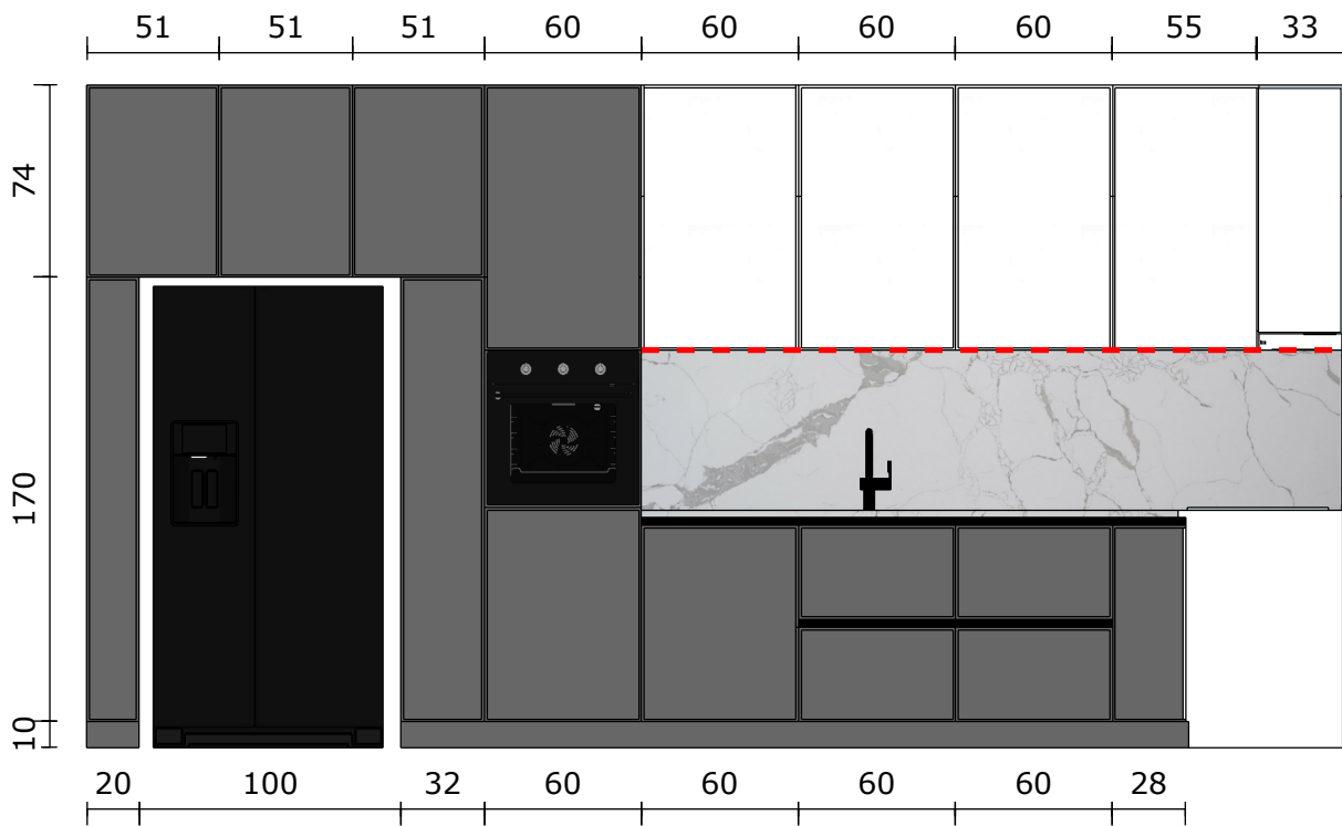
Pogled A_A
