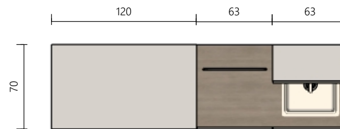
Tlocrt presjek A_A
