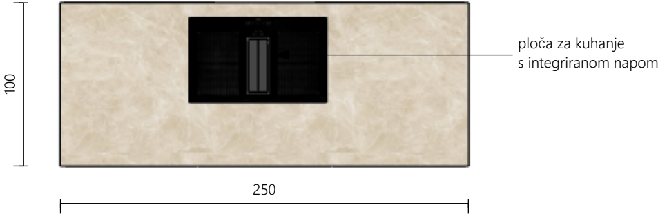
Tlocrt presjek BC
